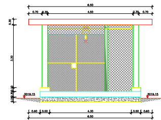
FACHADA LATERAL DERECHA ESCALA 1:50
