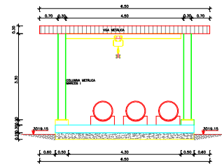
ESTRUCTURA DESINFECCION - CORTE ESCALA 1:50
