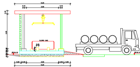
ESTRUCTURA DESINFECCION - CORTE ESCALA 1:50
