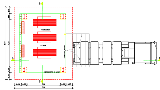
ESTRUCTURA DESINFECCION - PLANTA ESCALA 1:50
