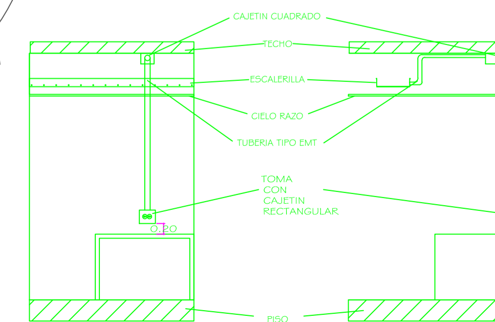
DETALLE DE TOMACORRIENTES CON TUBERIAS EMT SOBRE MESON ESCALA: 1:50
