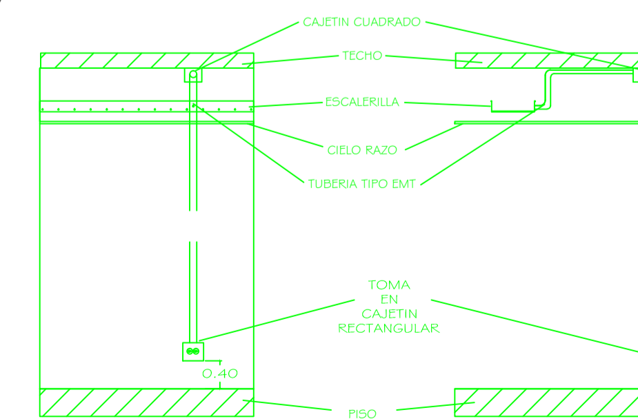
DETALLE DE TOMACORRIENTES CON TUBERIAS EMT ESCALA: 1 : 50
