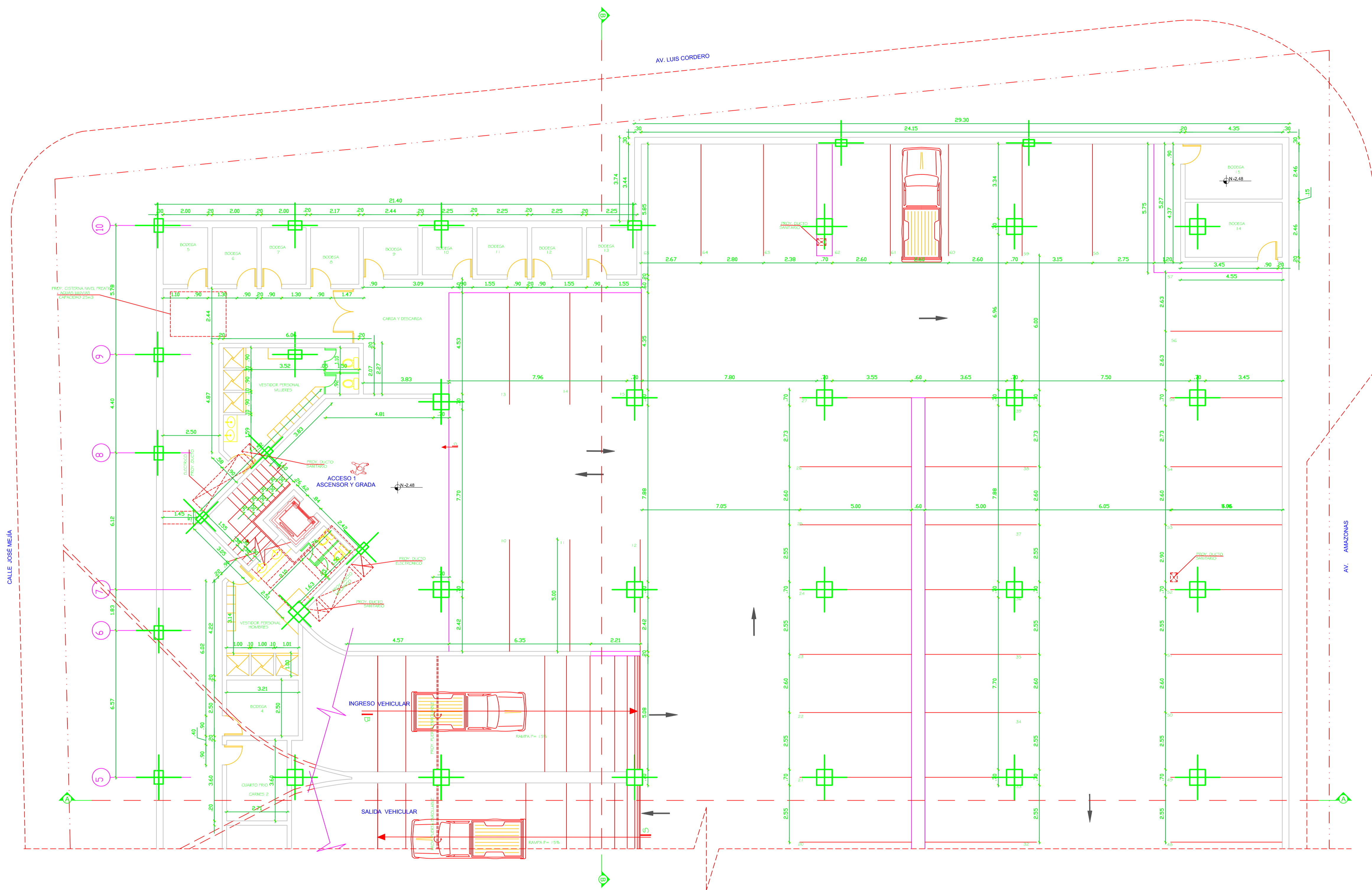
PLANTA SUBSUELO Nv. -2.66 ESCALA: 1:100
