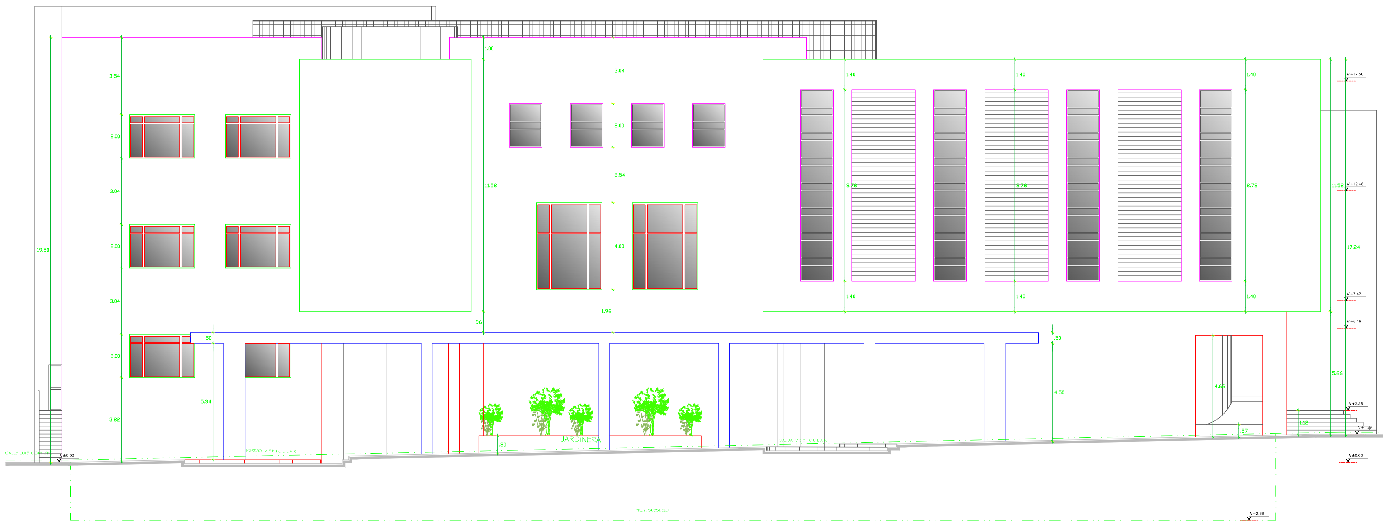
FACHADA CALLE JOSE MEJIA ESCALA: 1:100
