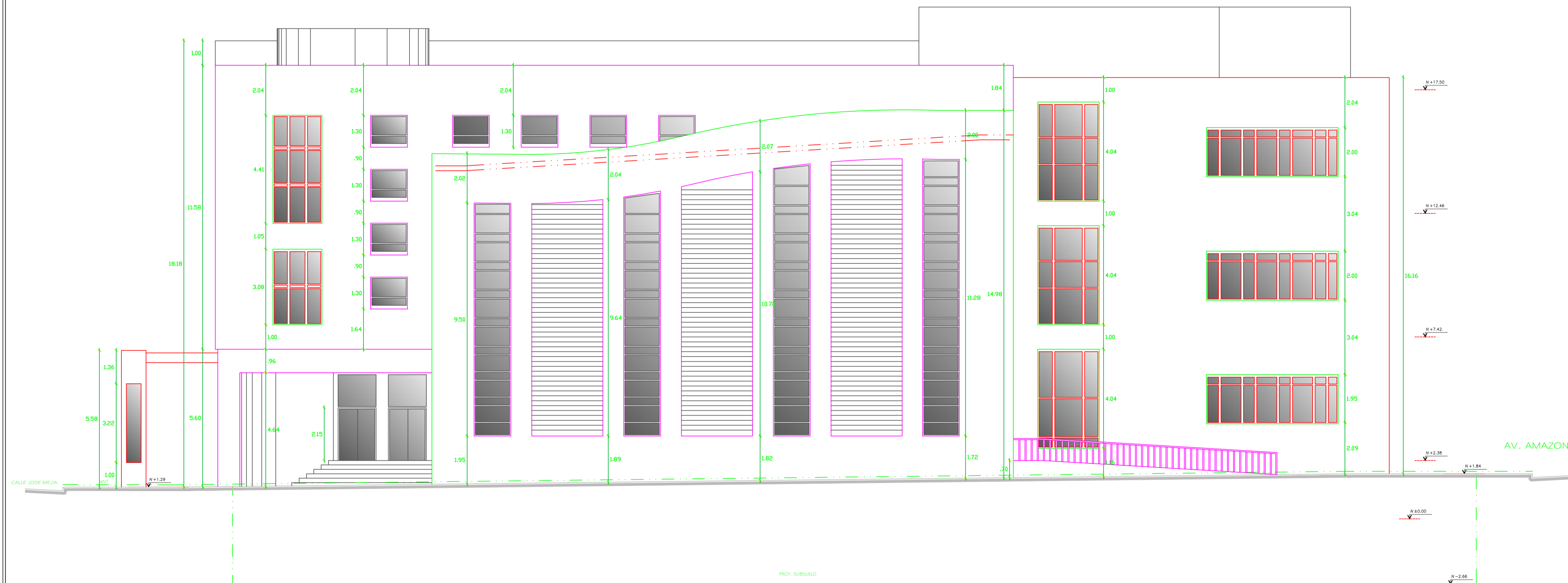
FACHADA CALLE 11 DE NOVIEMBRE ESCALA: 1:100
