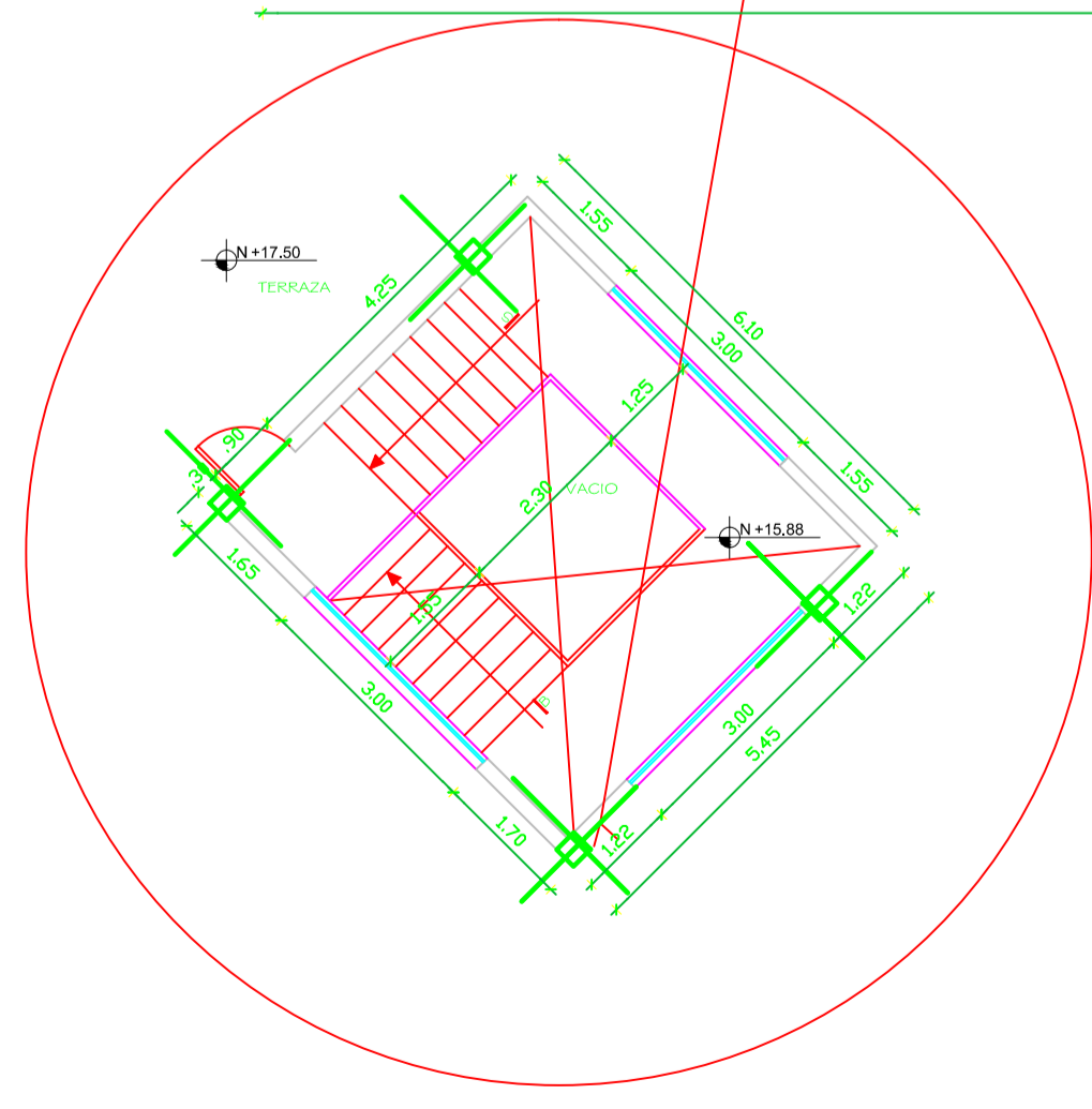
PLANTA NIVEL + 17.50 ESCALA: 1:100
