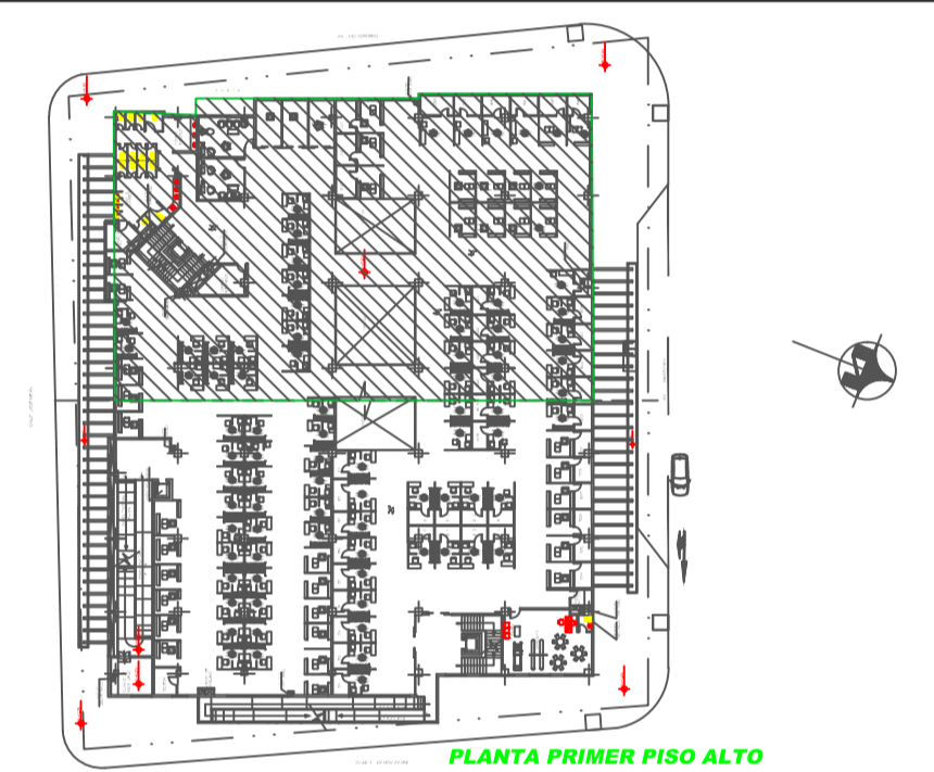
PLANTA PRIMER PISO ALTO
